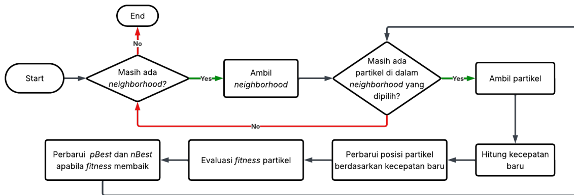
Gambar 3.18: Diagram alur pembaruan kecepatan dan posisi partikel PSO diskrit.
