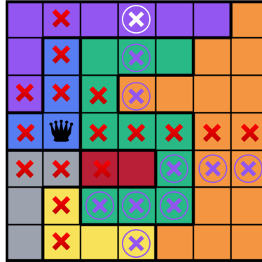
Gambar 3.12: Kondisi papan setelah propagasi AC-3 selesai.
