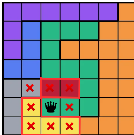
Gambar 2.5: Ilustrasi domain wipeout pada beberapa sektor warna sekaligus. Satu penempatan menteri secara bersamaan mengeliminasi seluruh kandidat sel pada dua sektor yang berdekatan, memperlihatkan bagaimana satu keputusan dapat memicu kegagalan berantai pada cabang pencarian.
