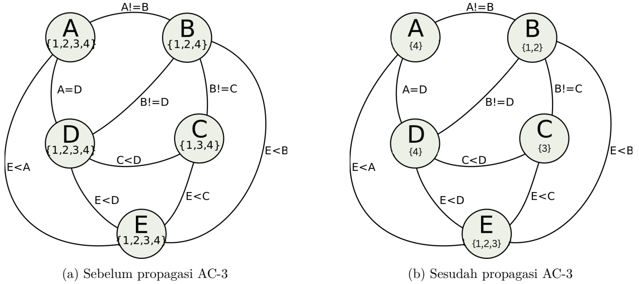
Gambar 2.7: Contoh propagasi AC-3 pada constraint graph dengan lima variabel. Sebelum propagasi (a), domain variabel masih lebar. Setelah AC-3 diterapkan (b), nilai-nilai yang tidak memiliki support dieliminasi, menghasilkan domain yang jauh lebih kecil.
