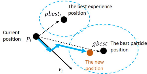
Gambar 2.8: Ilustrasi perpindahan satu partikel berdasarkan velocity baru yang dipengaruhi oleh personal best dan global best .
